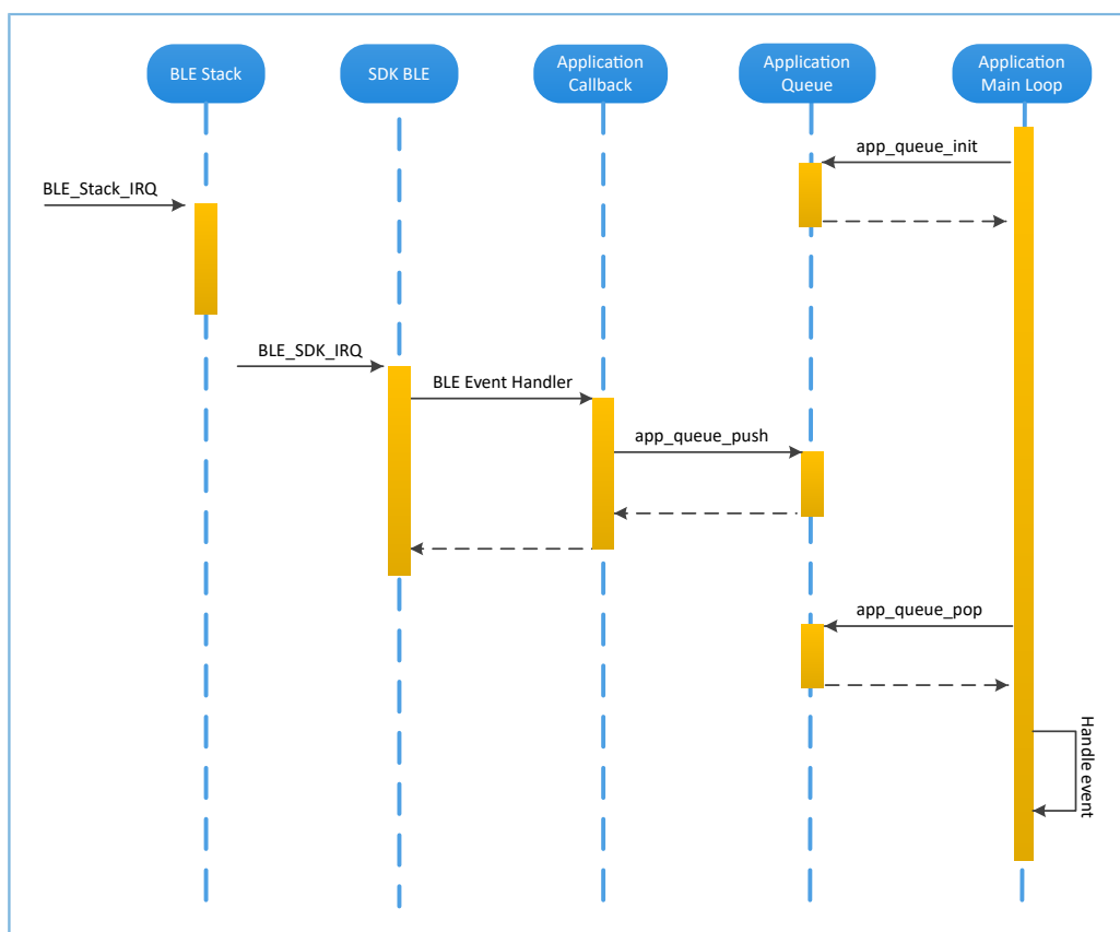
图 4-10 Non-OS system schedule
