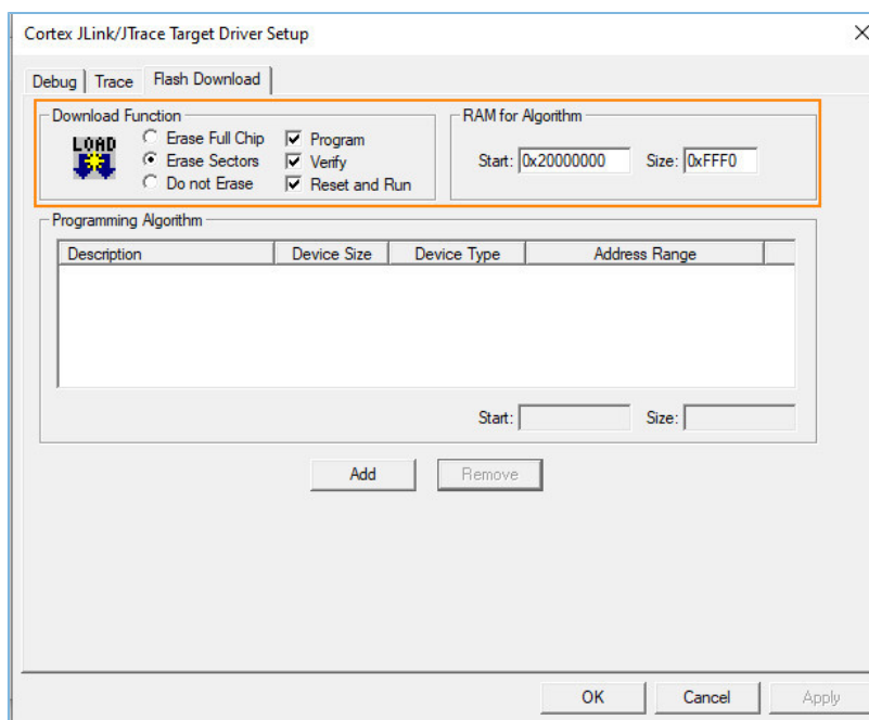
图 4-12 选择“Download Function”
