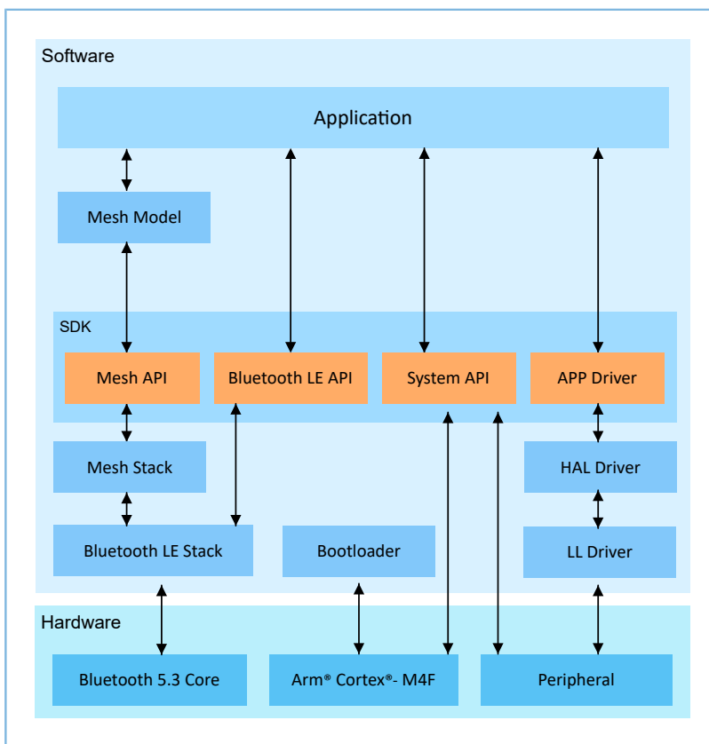
图 2-2 GR533x软件架构
