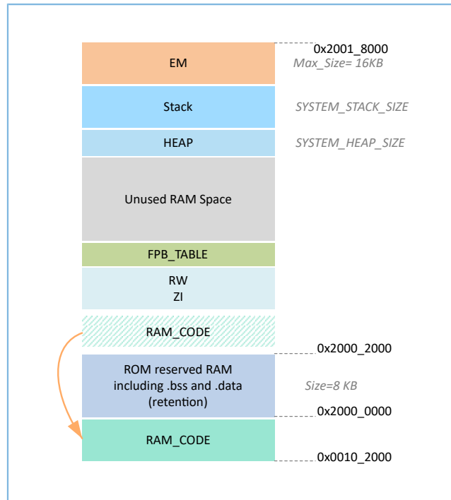
图 2-8 XIP模式的RAM（含Bluetooth LE工程）布局
