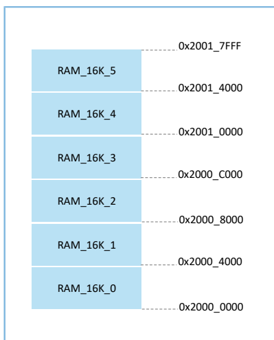
图 2-7 96 KB RAM存储布局
