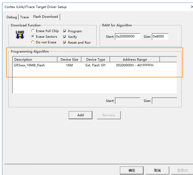
图 4-13 添加GR5xxx_16MB_Flash.FLM编程算法
