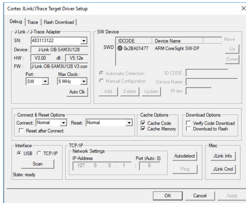
图 4-17 “Connect &amp; Reset Options” 配置
