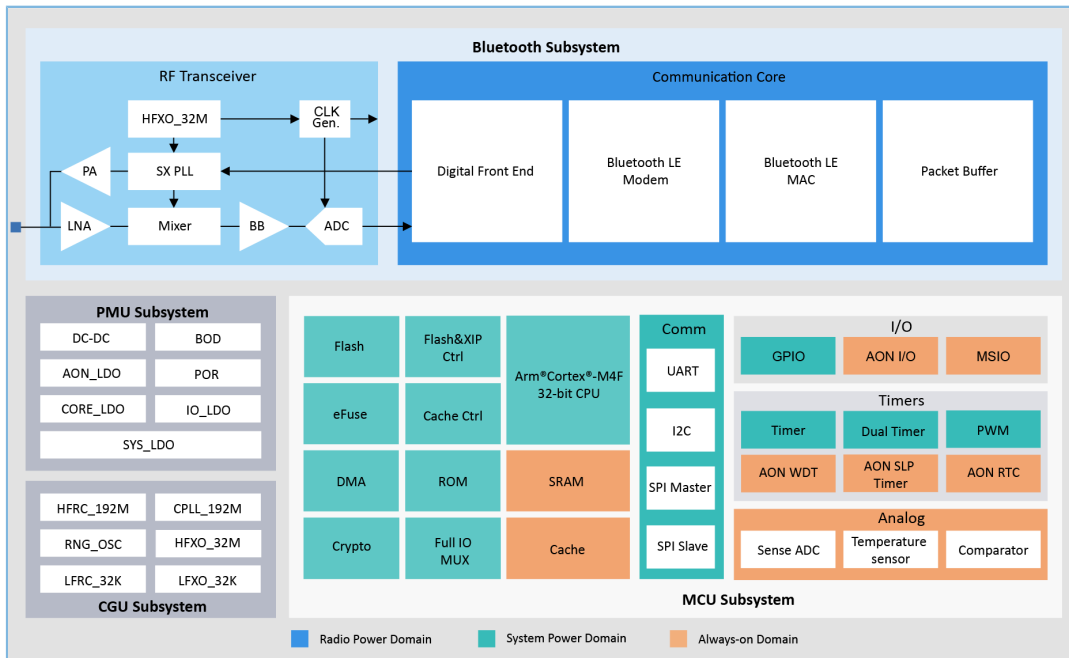
图 2-1 GR533x硬件框图
