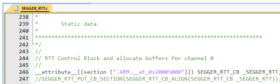
图 4-18 创建RTT Control Block并置于地址0x20005000处
