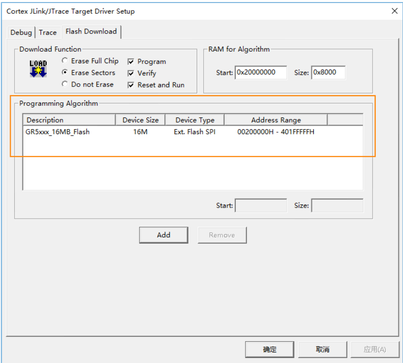
图 4-13 添加GR5xxx_16MB_Flash.FLM编程算法
