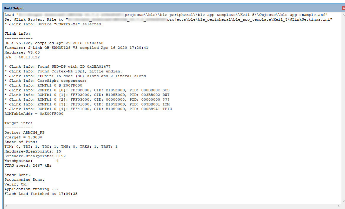
图 4-15 下载结果
