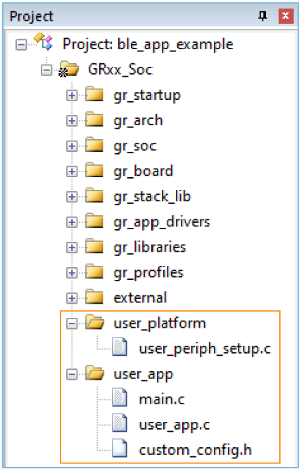
图 4-6 user_groups
