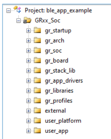
图 4-4 ble_app_example groups
