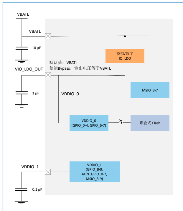
图 3-7 VIO_LDO_OUT与I/O电压域关系示意图
