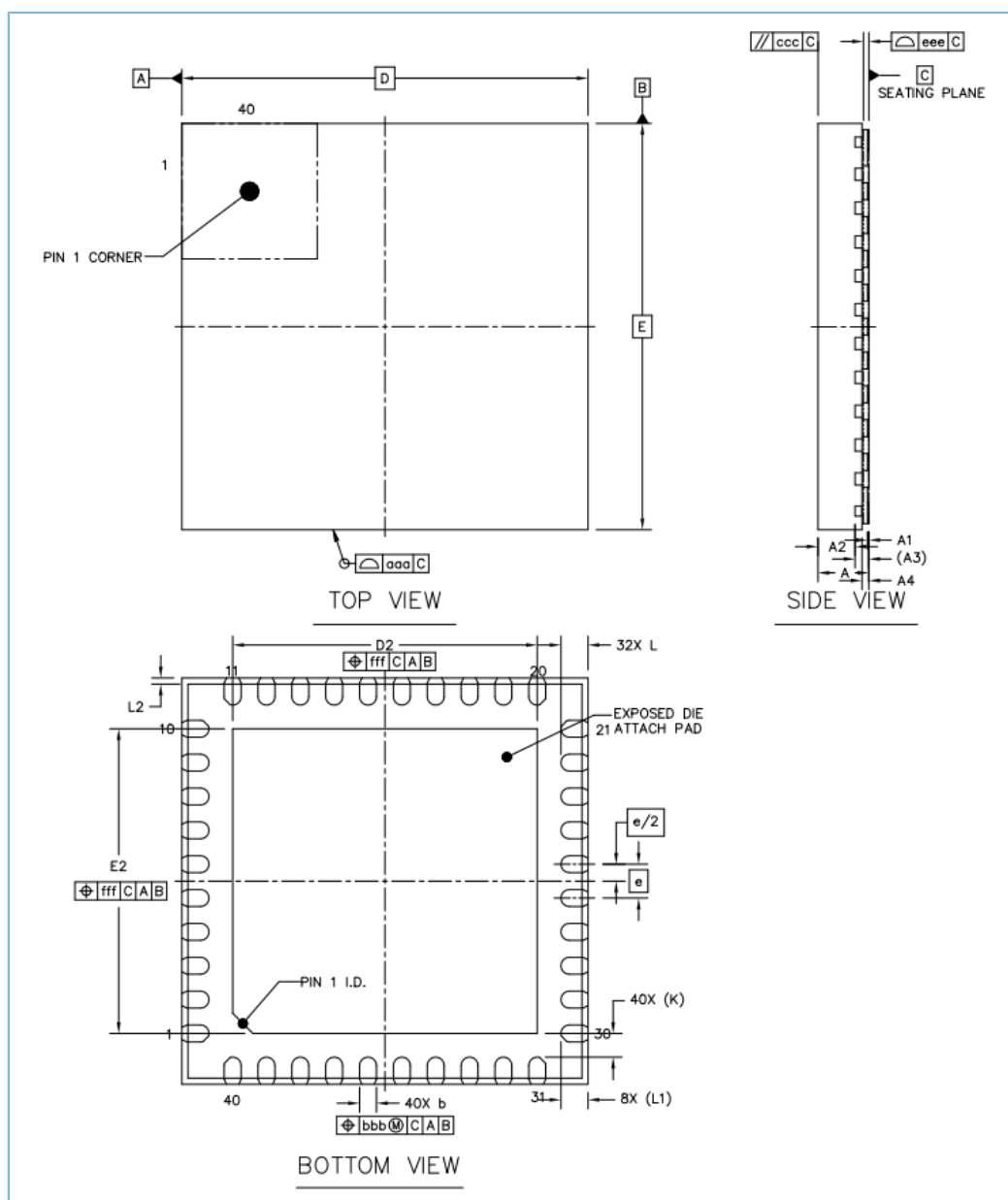
图 6-1 Wettable QFN40封装外形尺寸
