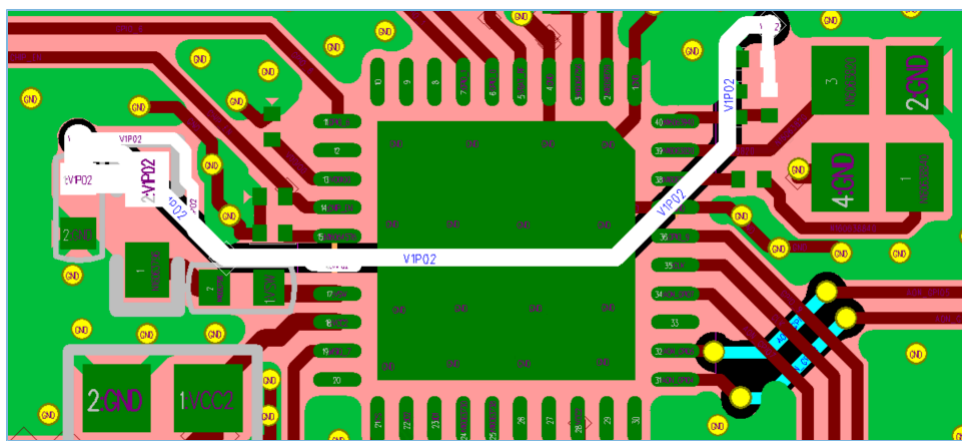
图 3-15 RF输入电源参考布局和走线
