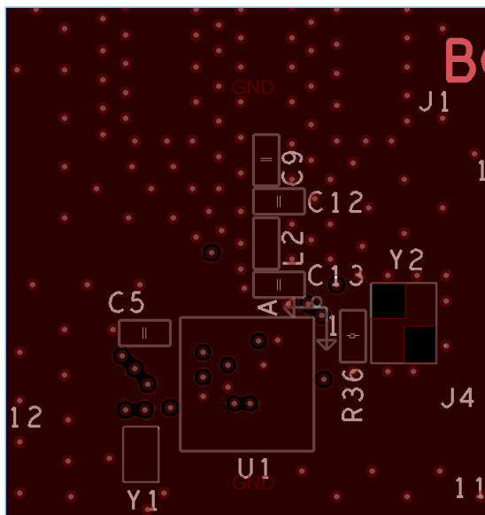
图 4-17 L2层设计
