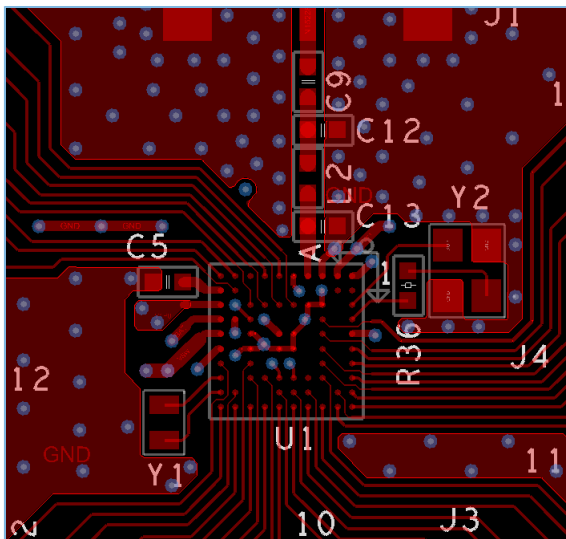
图 4-16 TOP层设计
