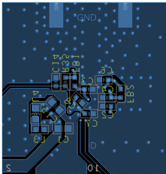
图 4-19 BOTTOM层设计
