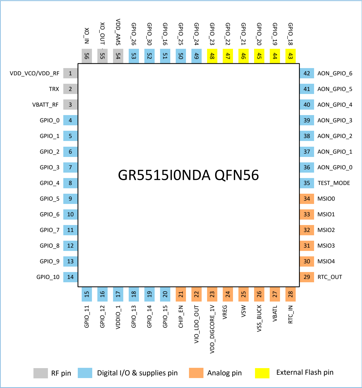
图 2-2 GR5515I0NDA QFN56封装引脚排列
