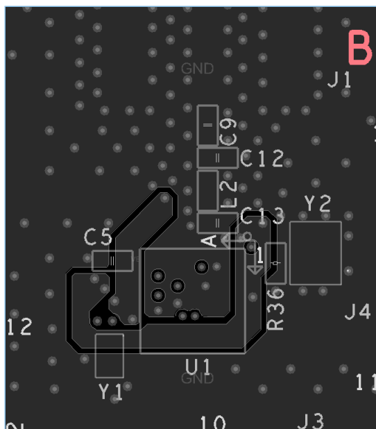
图 4-18 L3层设计
