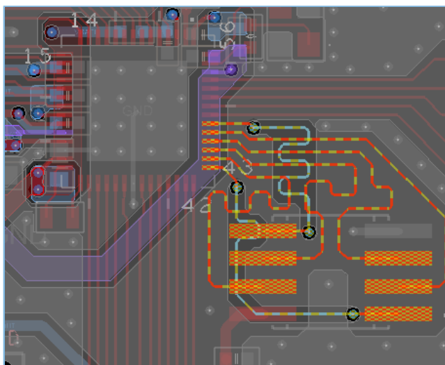
图 4-15 GR5515I0NDA PCB布局参考设计
