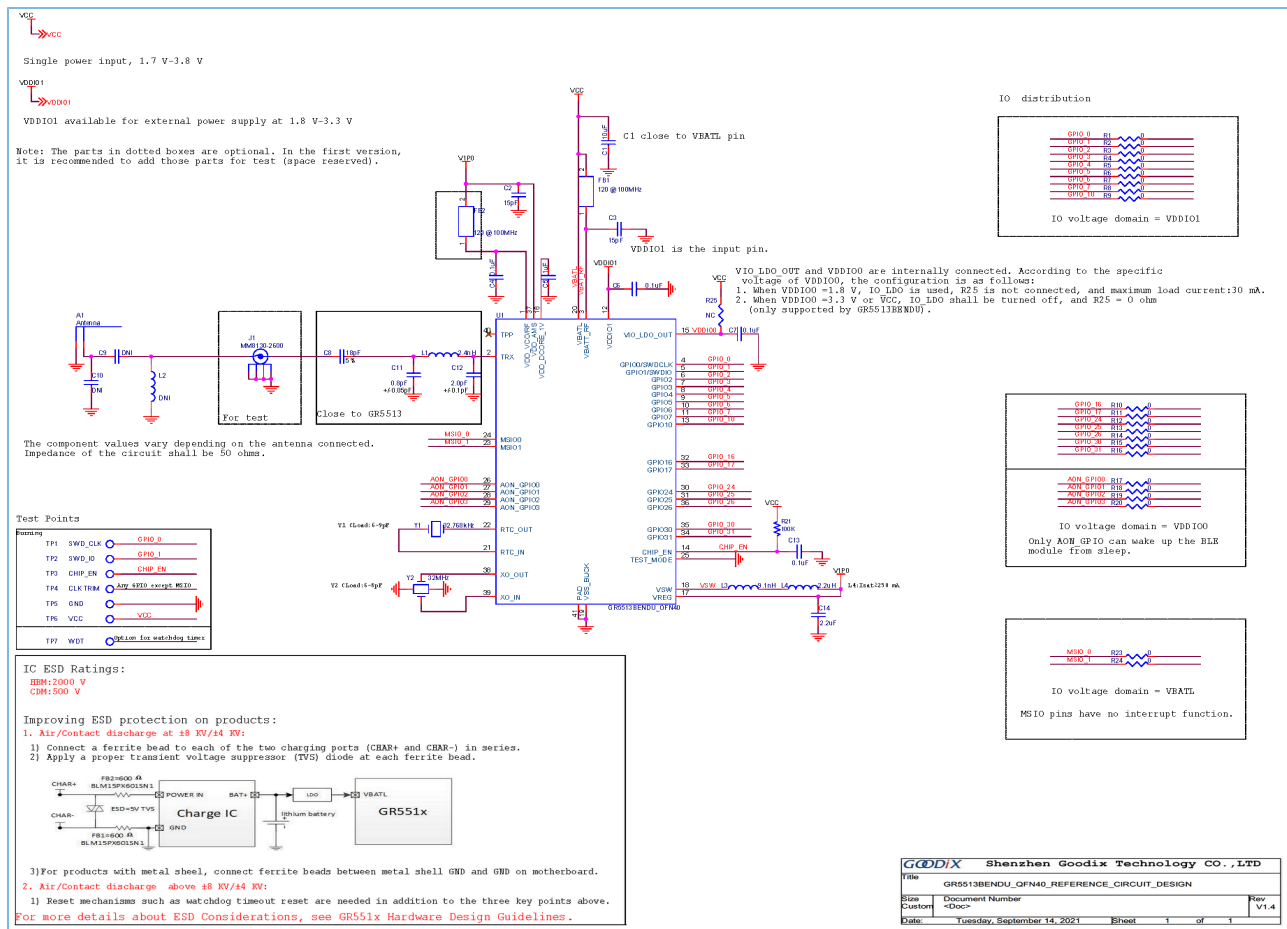
图 4-7 GR5513BENDU QFN40封装的参考电路
