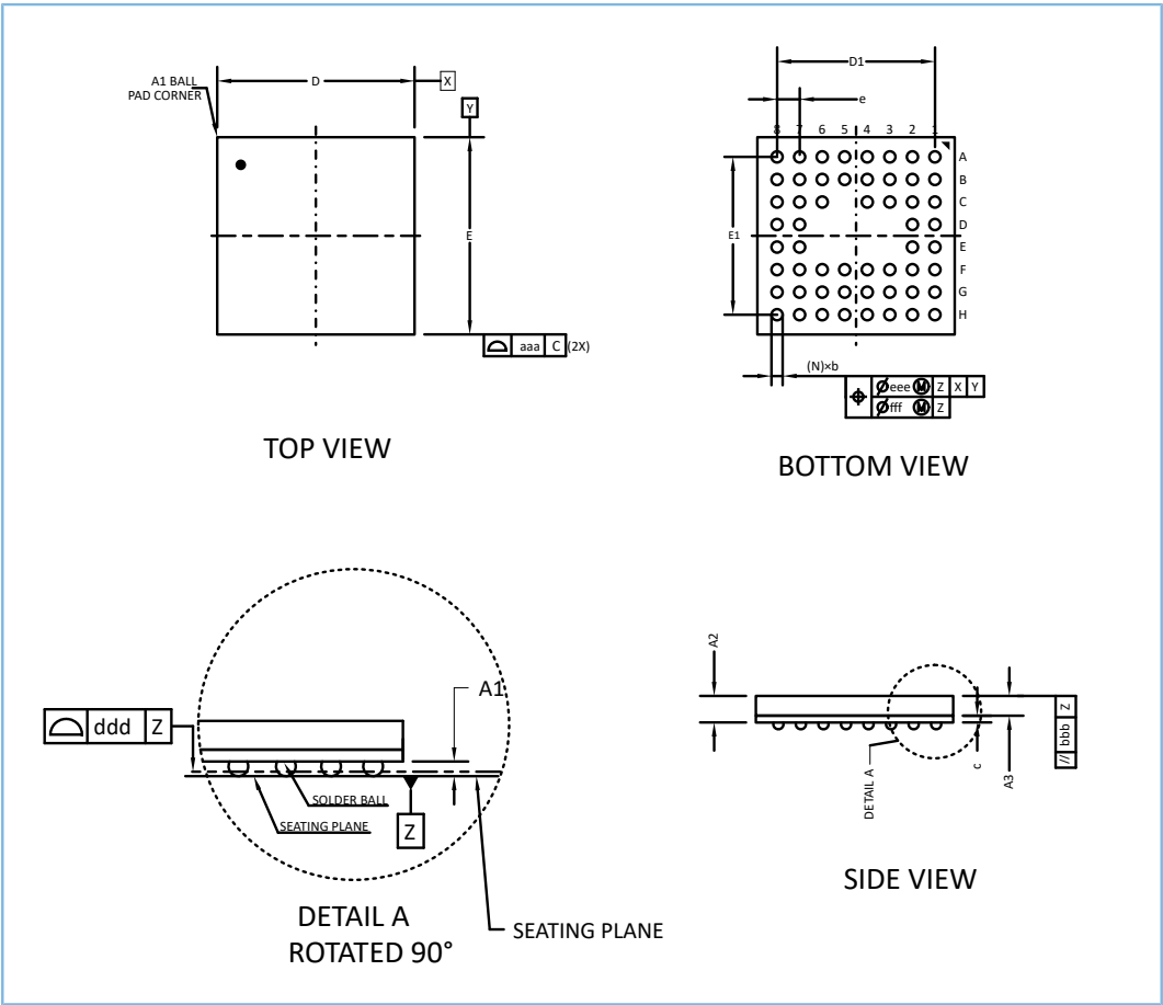
图 7-5 BGA55 封装外形尺寸
