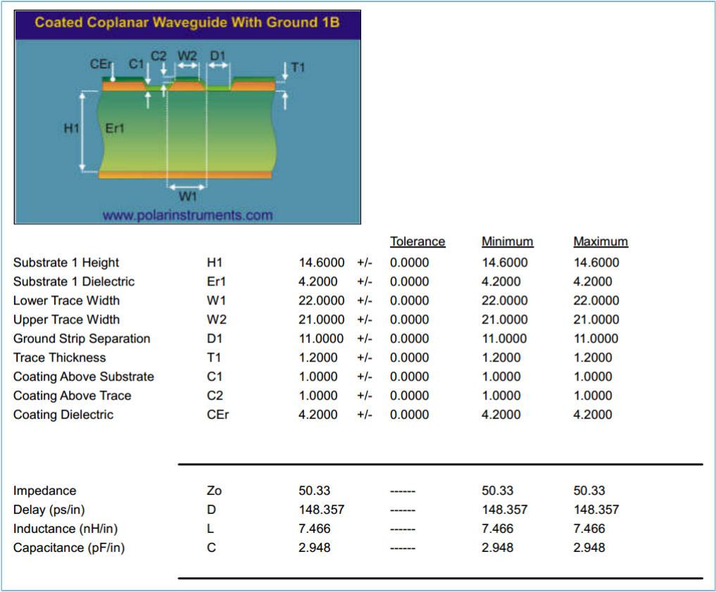
图 4-8 阻抗控制叠层设计
