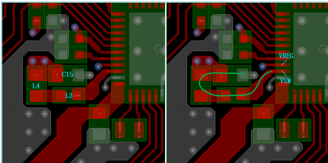
图 3-7 DC-DC电源输出参考布局和走线
