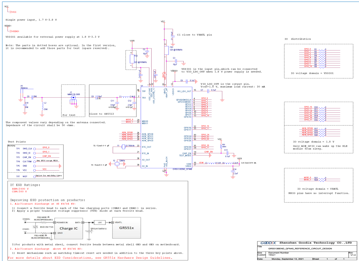
图 4-6 GR5513BEND QFN40封装的参考电路
