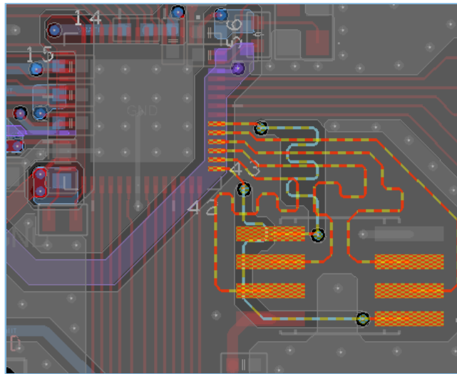
图 4-14 GR5515I0NDA PCB布局参考设计
