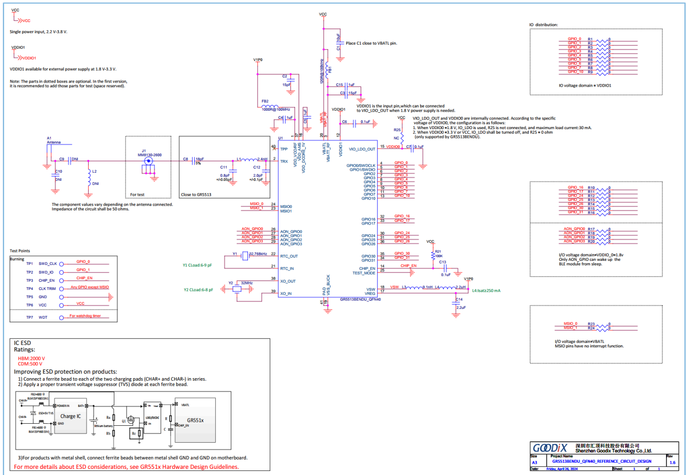
图 4-6 GR5513BENDU QFN40封装的参考电路
