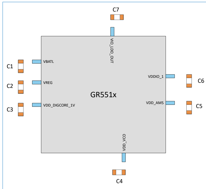
图 3-20 电源滤波电容布局示意图
