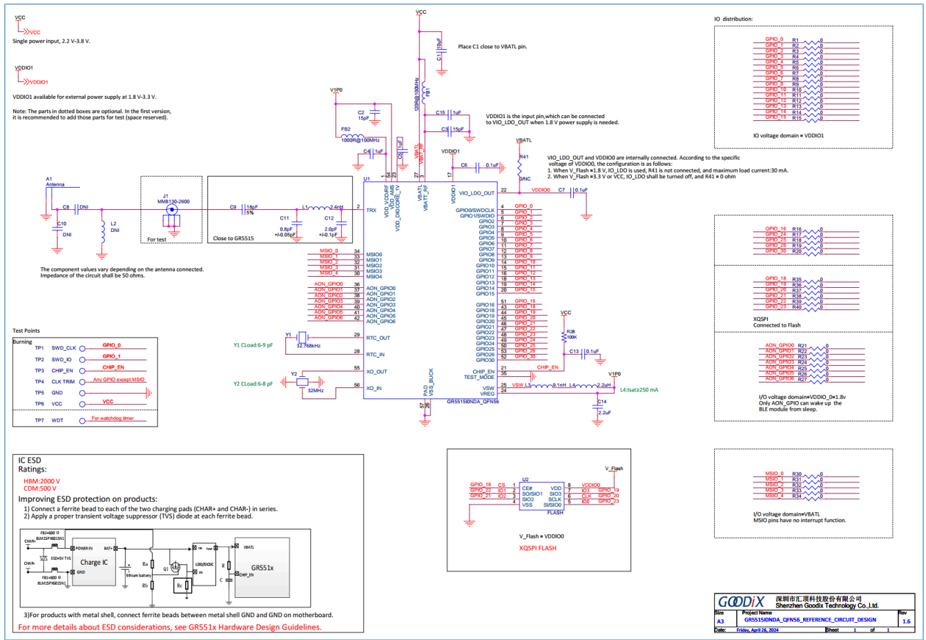
图 4-3 GR5515IONDA QFN56封装的参考电路
