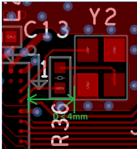
图 3-15 GR5515RGBD PCB参考时钟布局
