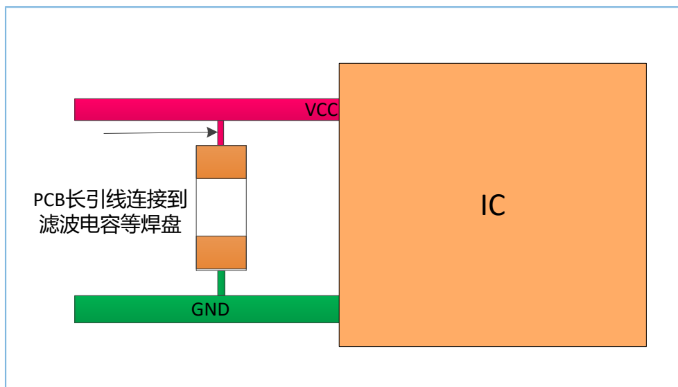
图 3-24 错误的电容或ESD防护器件走线
