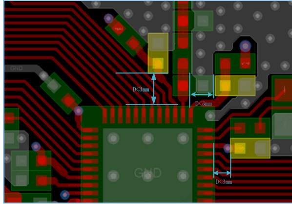
图 3-13 RF输入电源参考布局和走线
