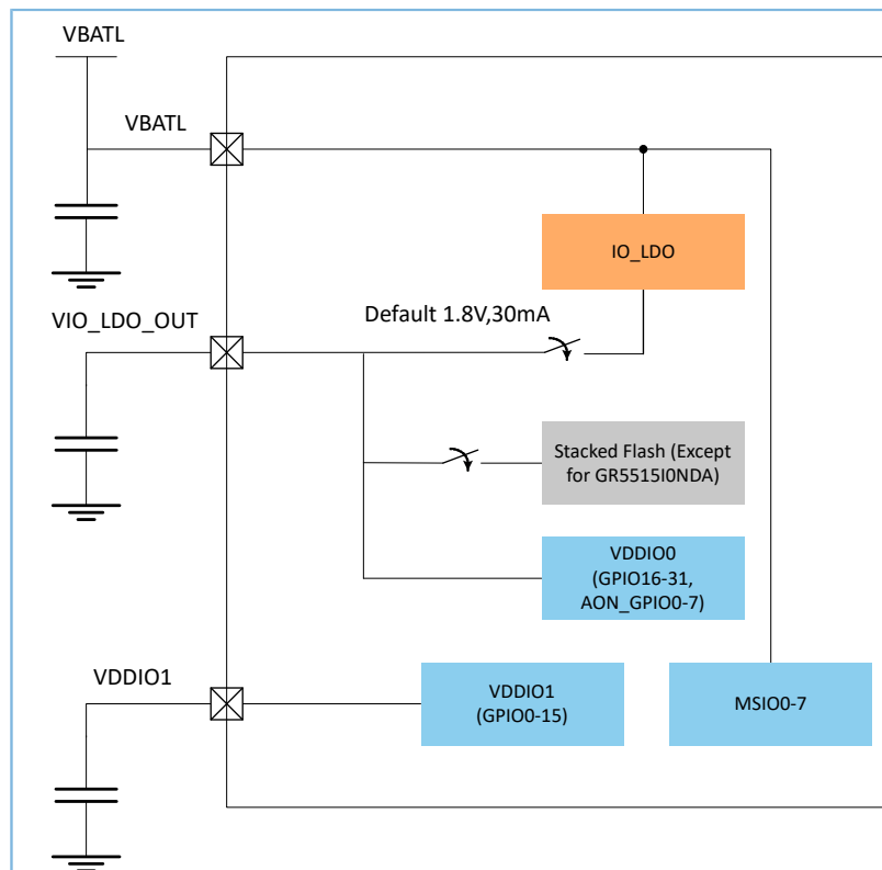
图 3-8 VIO_LDO_OUT与IO电压域关系示意图
