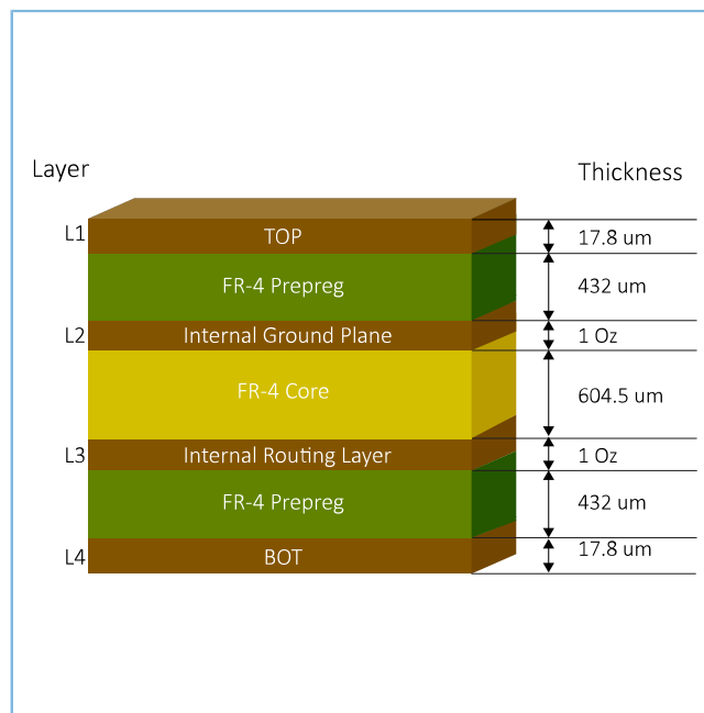
图 3-11 GR551x PCB参考叠层结构
