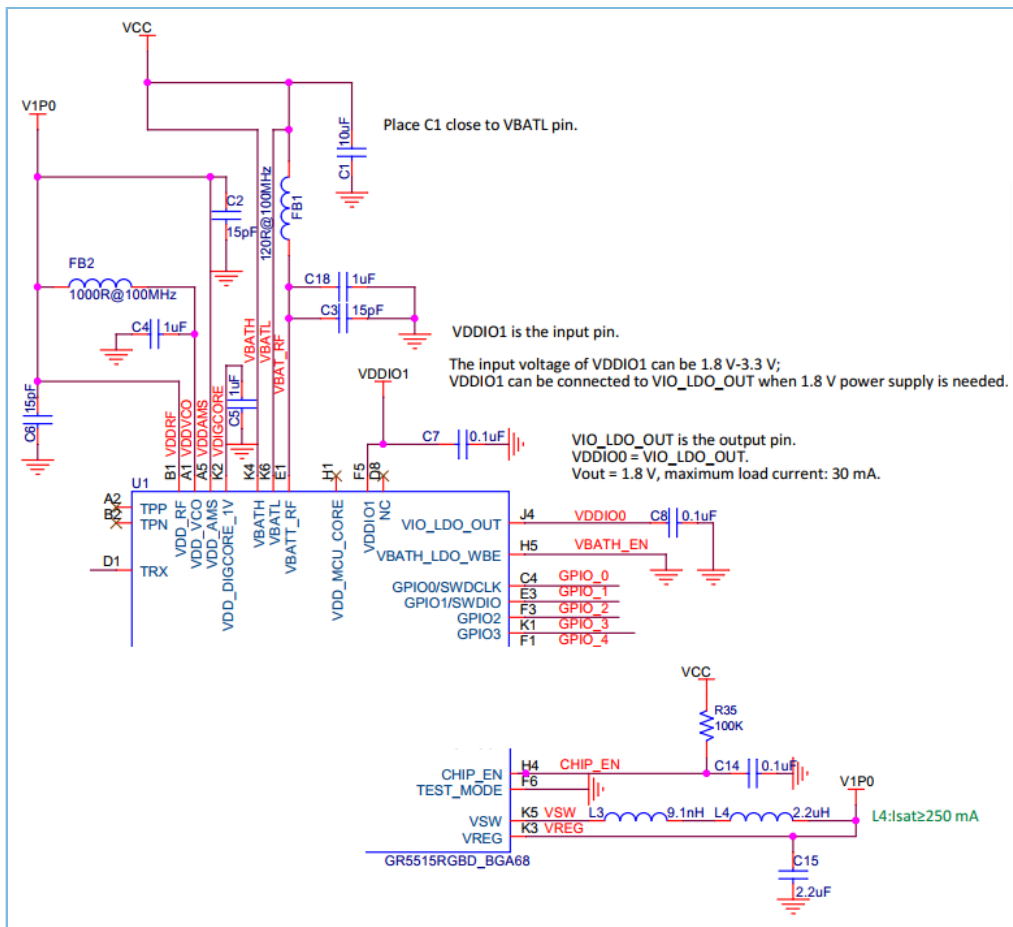
图 3-7 GR551x 电源原理图
