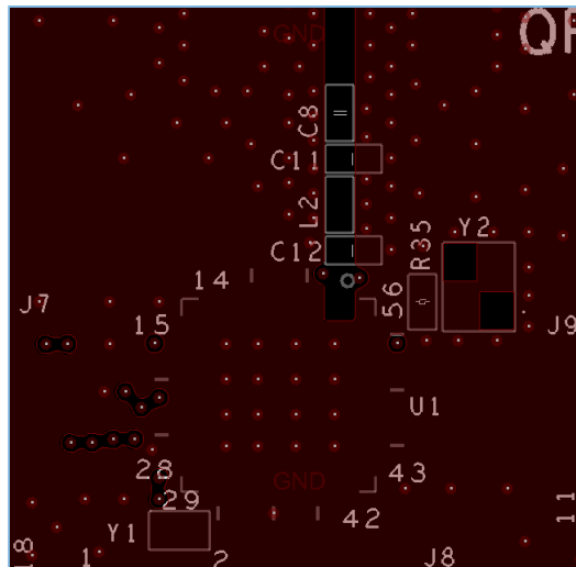
图 4-9 L2层设计
