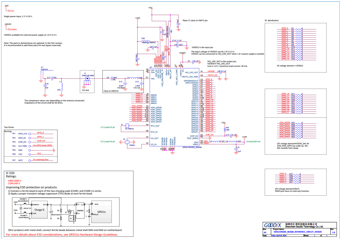
图 4-4 GR5515RGBD BGA68封装的参考电路
