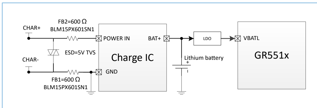
图 3-18 电源充电接口ESD处理
