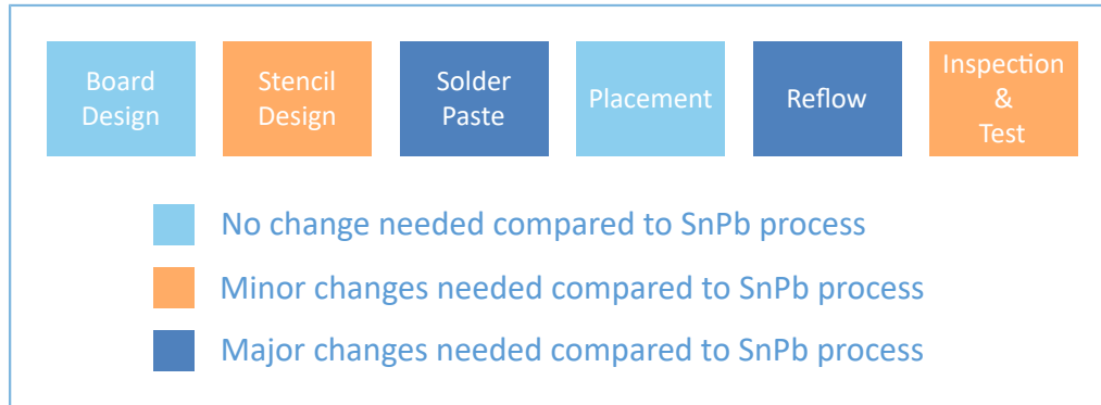
图 7-8 SMT 印刷流程
