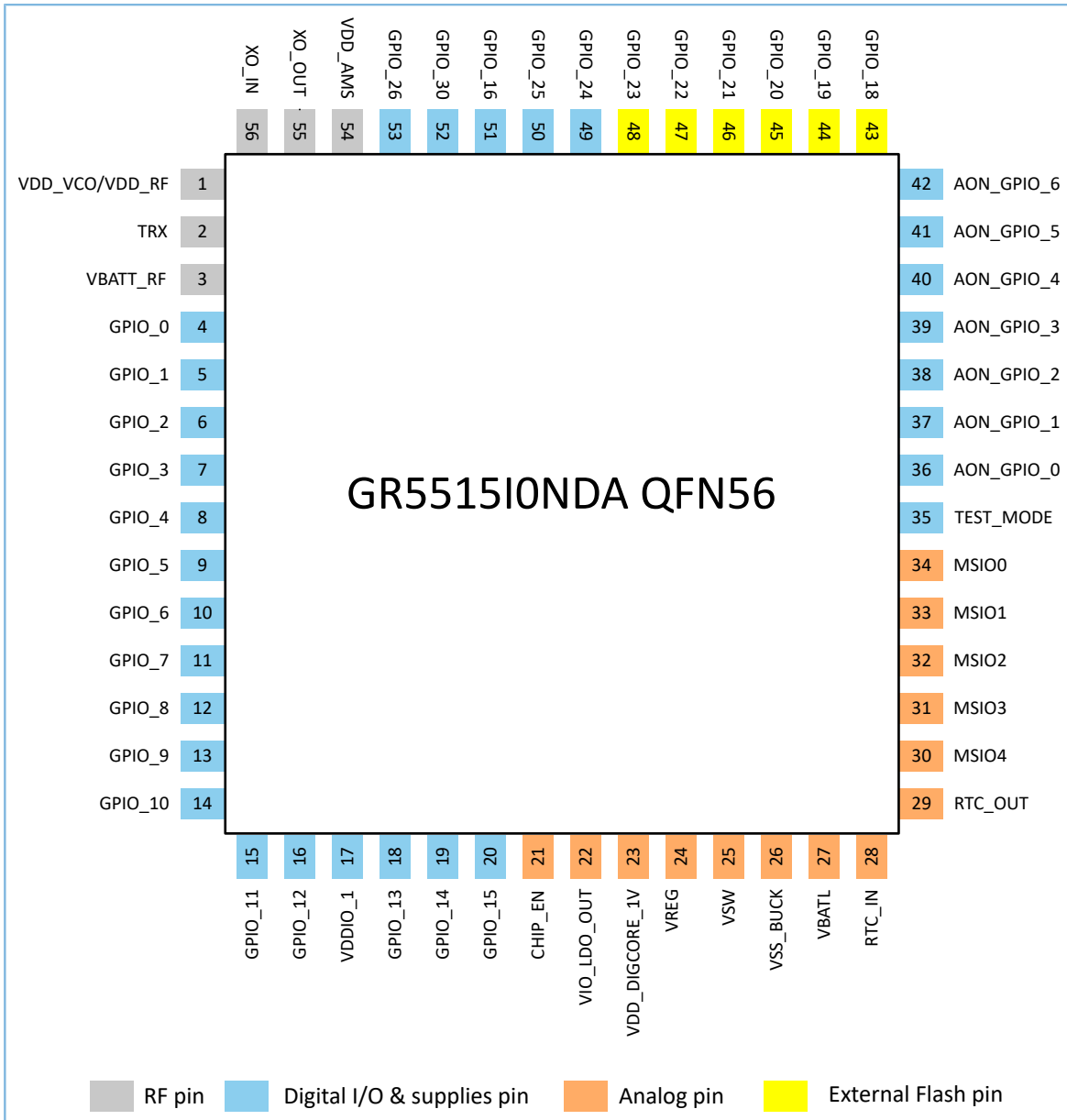
图 2-2 GR5515IONDA QFN56封装引脚排列
