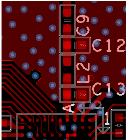
图 3-17 射频端口的PCB布局
