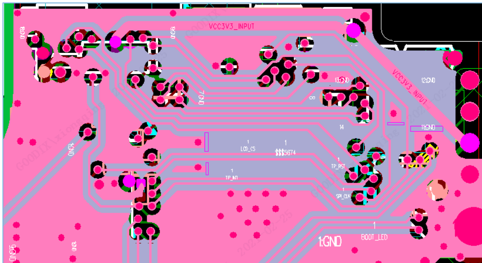
图 3-22 正确的IO走线处理
