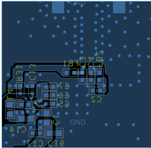
图 4-11 BOTTOM层设计
