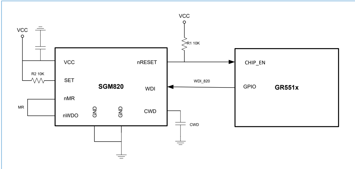
图 3-19 硬件看门狗参考设计电路
