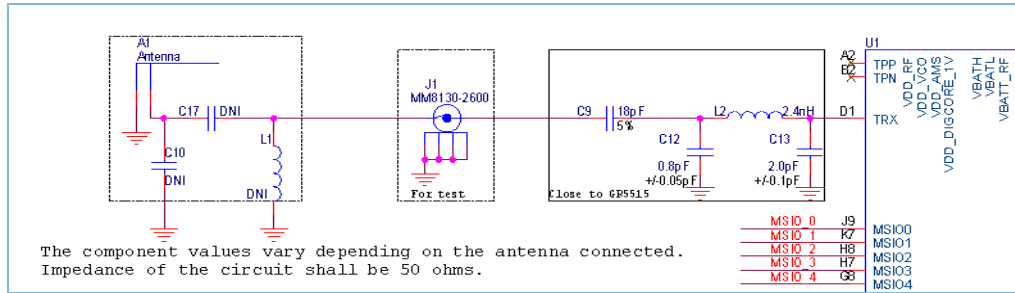
图 3-10 射频电路原理图
