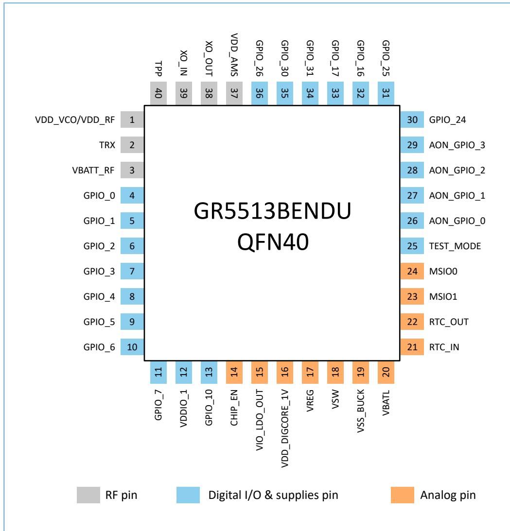
图 2-5 GR5513BENDU QFN40封装引脚排列
