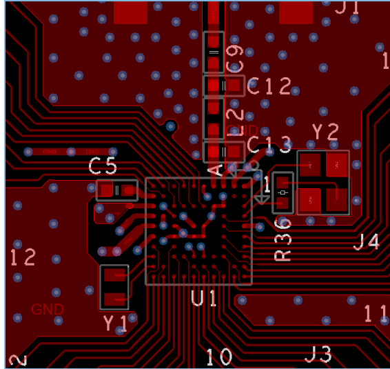
图 4-15 TOP层设计
