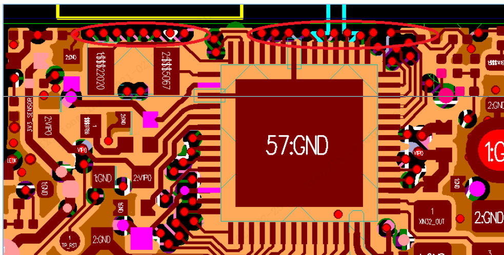
图 3-21 错误的IO走线处理（未包地）
