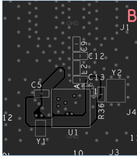
图 4-17 L3层设计
