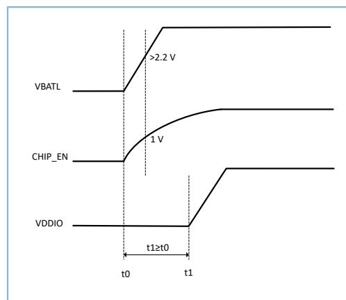
图 3-2 上电时序
