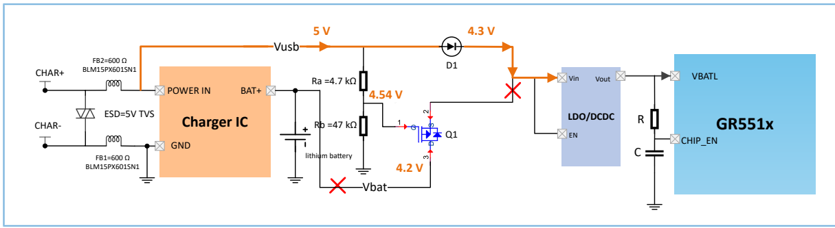
图 3-6 充电或充满电时的供电路径
