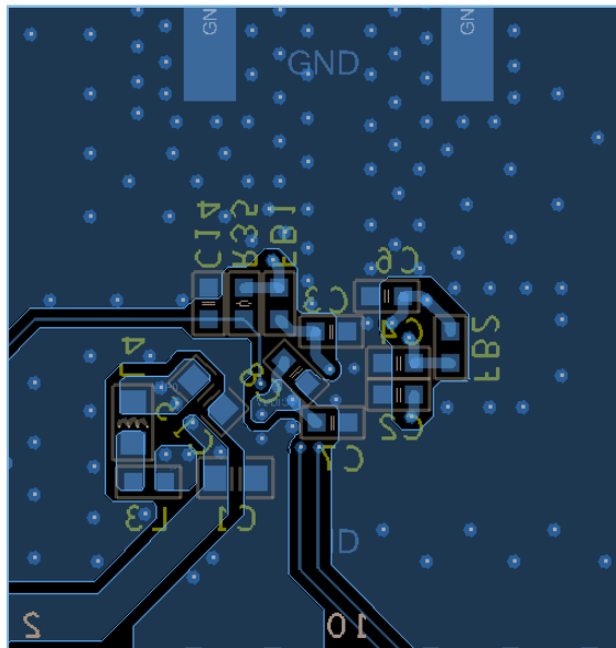
图 4-18 BOTTOM层设计
