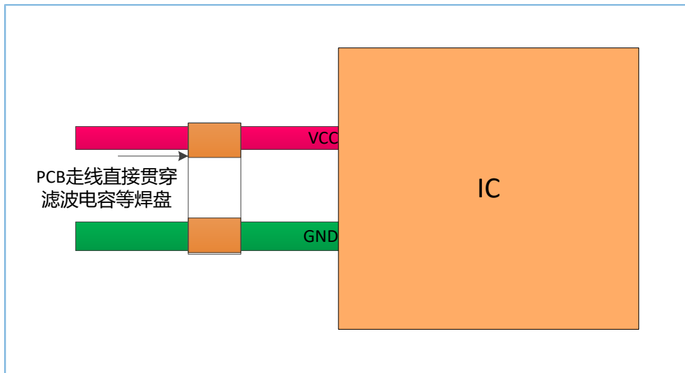
图 3-23 正确的电容或ESD防护器件走线
