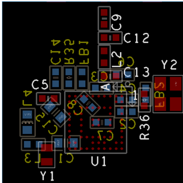
图 3-14 GR5515RGBD PCB参考电源布局
