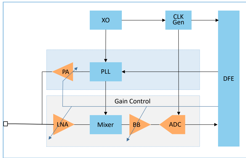
图 3-9 GR551x收发器框图
