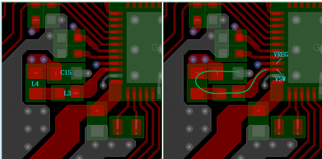
图 3-12 DC-DC电源输出参考布局和走线
