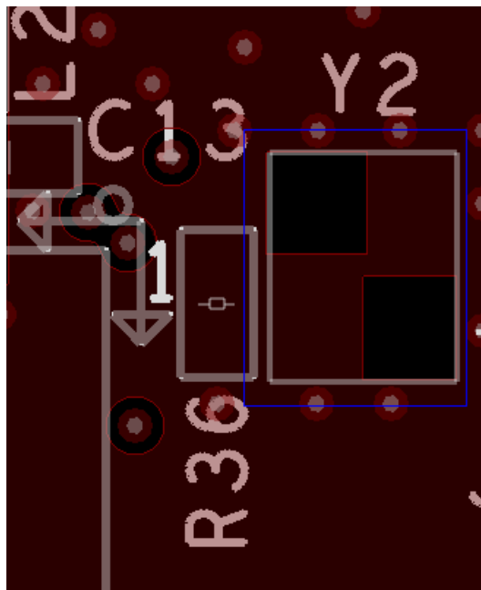
图 3-16 GR5515RGBD PCB晶振开窗处理
