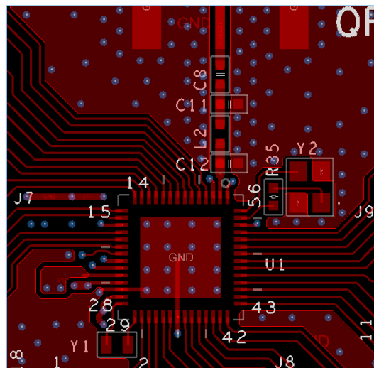
图 4-8 TOP层设计
