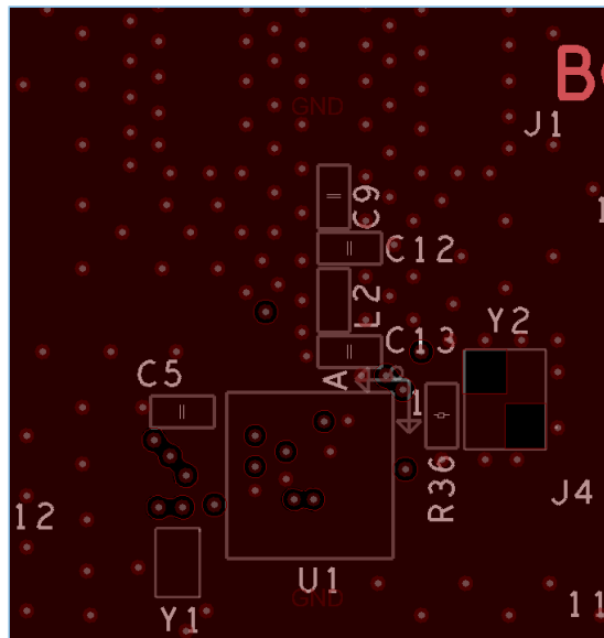
图 4-16 L2层设计
