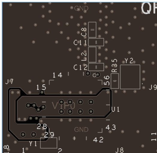
图 4-10 L3层设计
