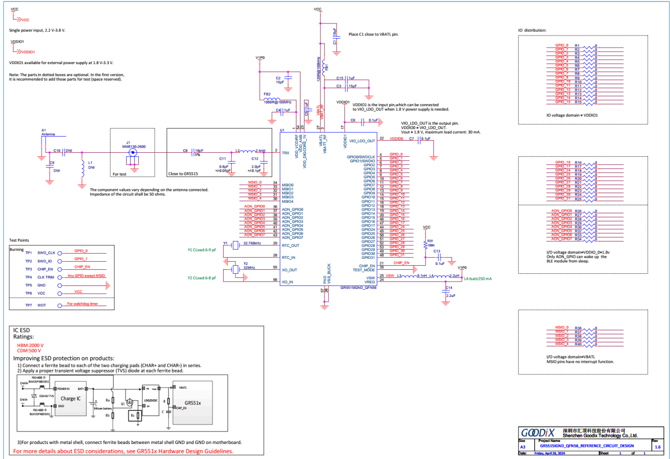
图 4-1 GR5515IGND QFN56封装的参考电路
