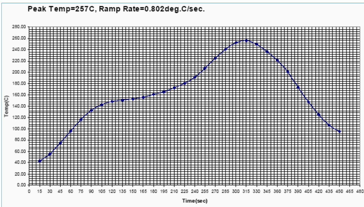
图 7-10 峰值温度为257°C的回流曲线示例
