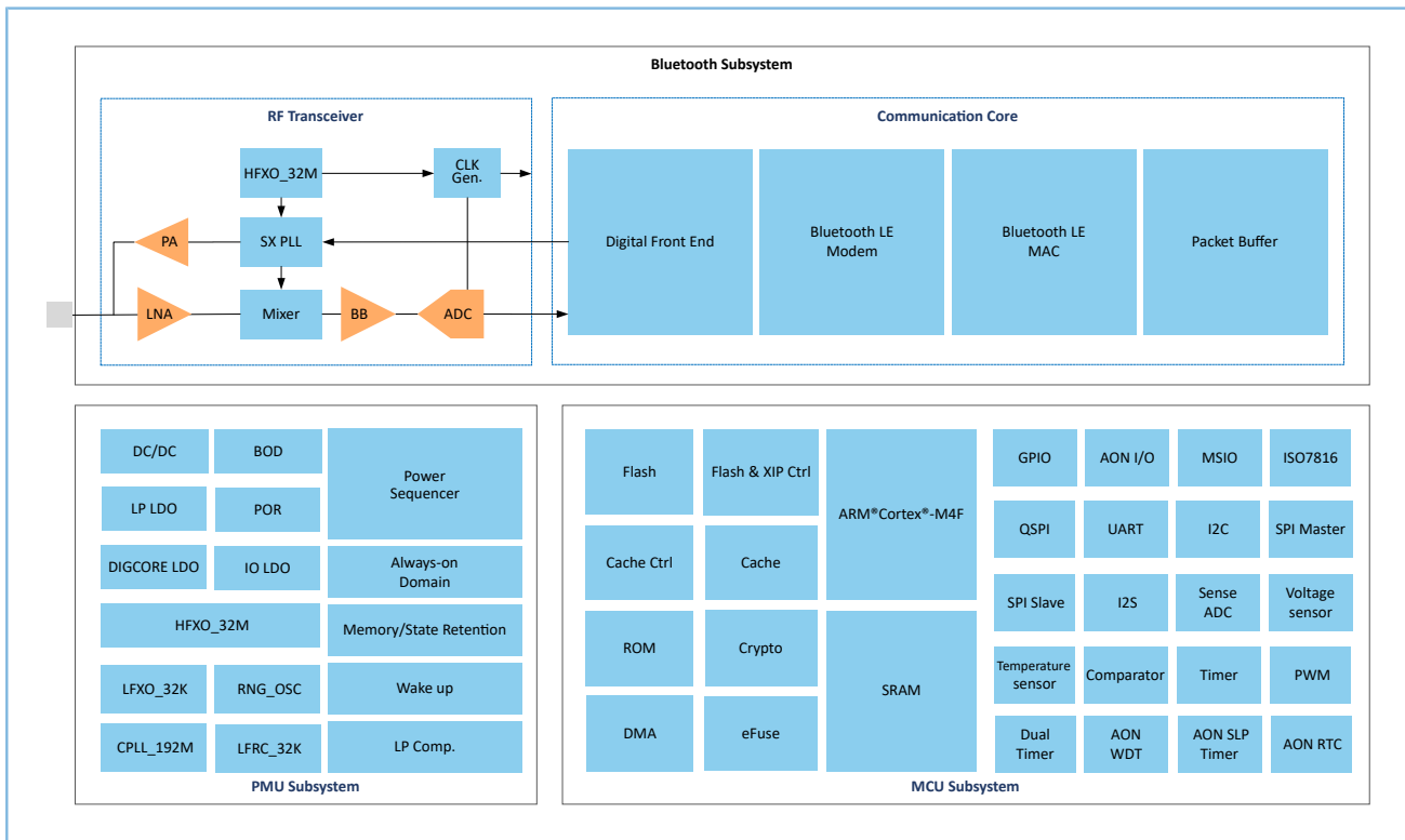
图 1-1 GR551x系统框图
