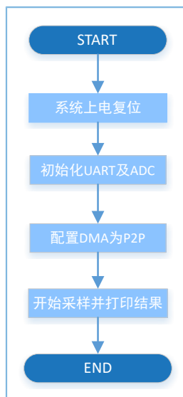
图 3-3 ADC DMA UART示例工程流程图
