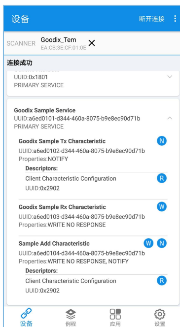
图 4-2 查看自定义Sample Service特性值
