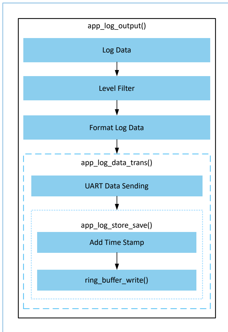
图 4-1 APP Log日志输出函数调用关系
