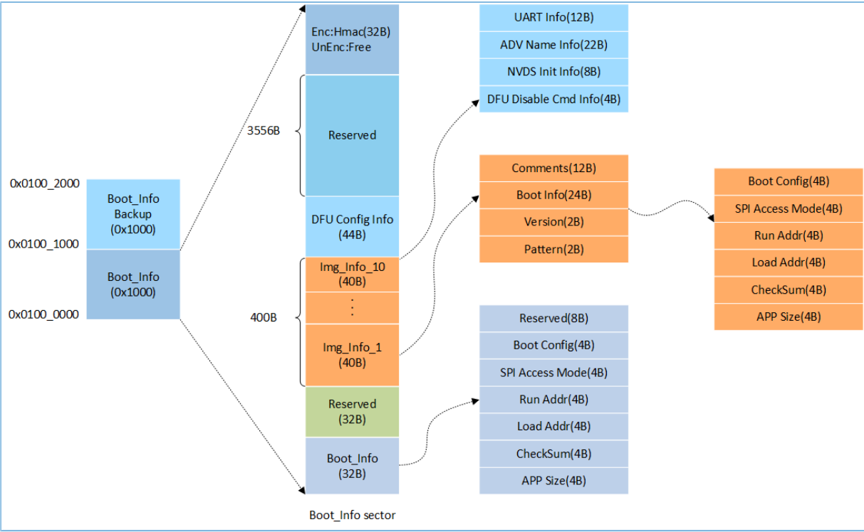
图 2-3 Flash中Boot_Info的结构
