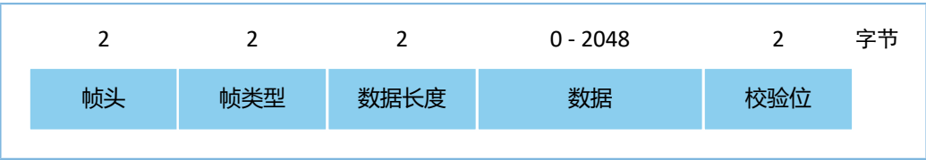
图 2-4 帧结构
