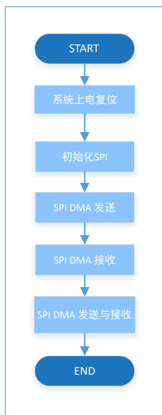
图 3-28 SPIM DMA示例流程图
