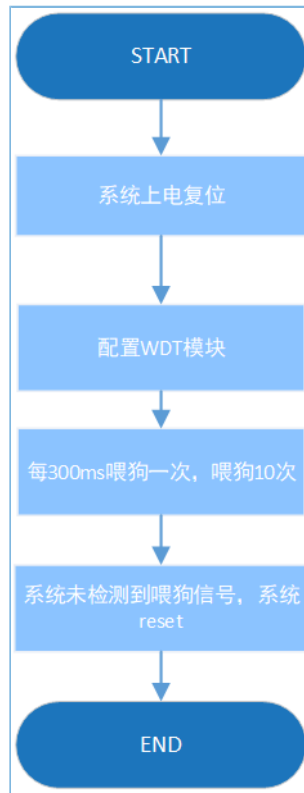
图 3-42 WDT Reset工程流程图
