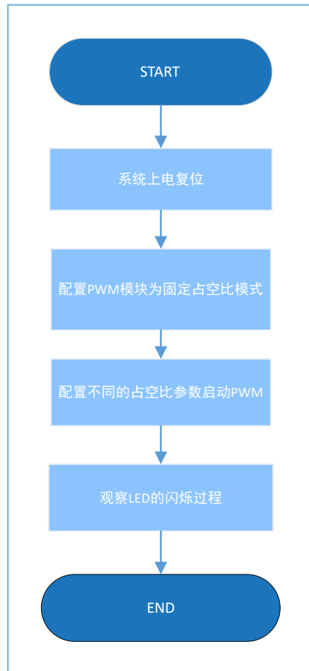
图 3-23 PWM Flicker示例工程流程图
