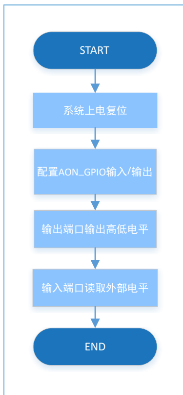
图 3-7 AON_GPIO Input & Output示例工程流程图
