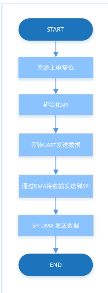
图 3-29 SPI DMA UART示例流程图
