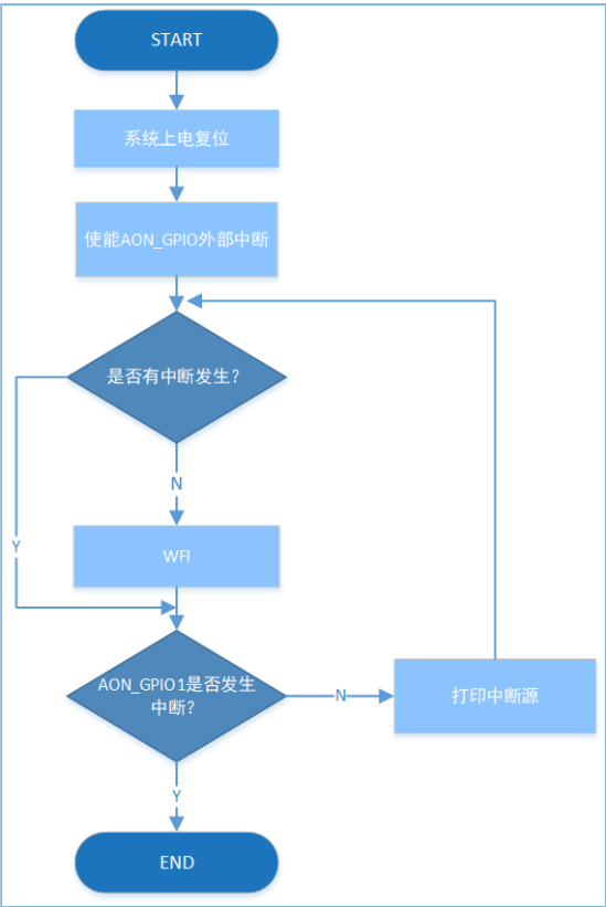
图 3-9 AON_GPIO Wakeup 示例工程流程图（WFI/WFE）
