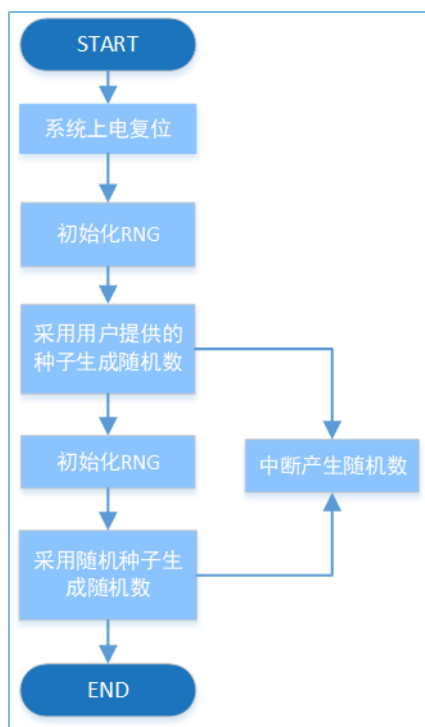
图 3-24 RNG Interrupt示例工程流程图
