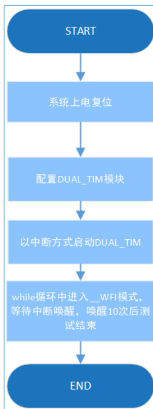
图 3-41 Timer Wakeup工程流程图
