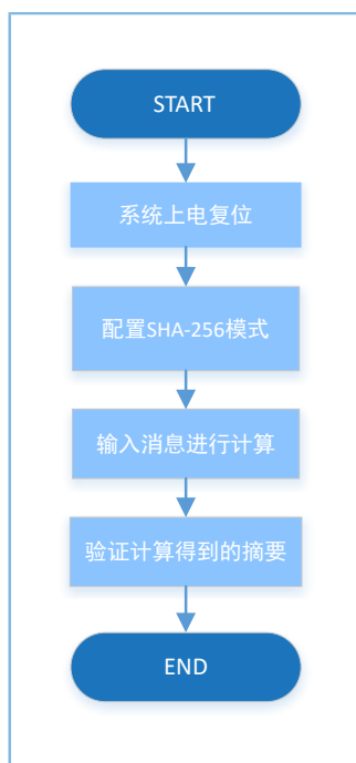
图 3-13 HMAC示例工程流程图（SHA-256）
