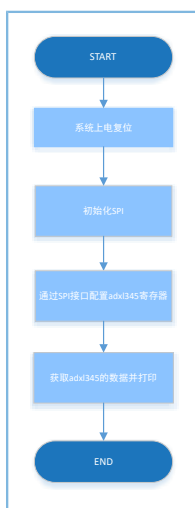
图 3-30 SPIM ADXL345示例流程图
