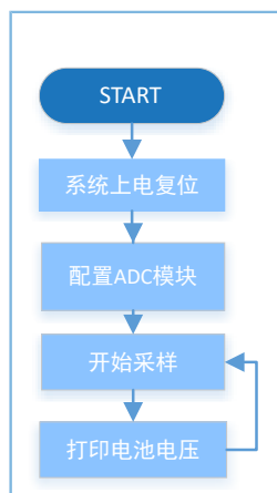
图 3-4 ADC Battery示例工程流程图
