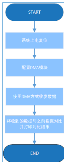
图 3-35 DMA Memory to Memory工程流程图
