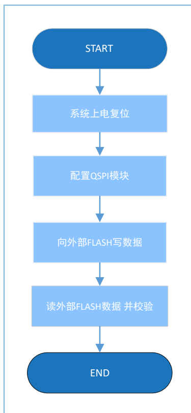
图 3-36 QSPI Flash工程流程图
