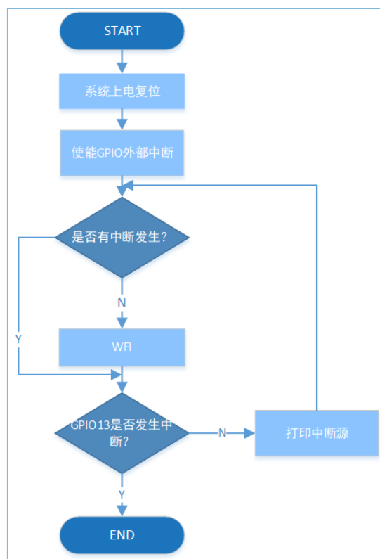
图 3-12 GPIO Wakeup示例工程流程图（WFI/WFE）
