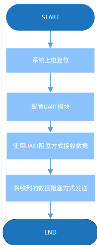
图 3-34 UART TX & RX工程流程图
