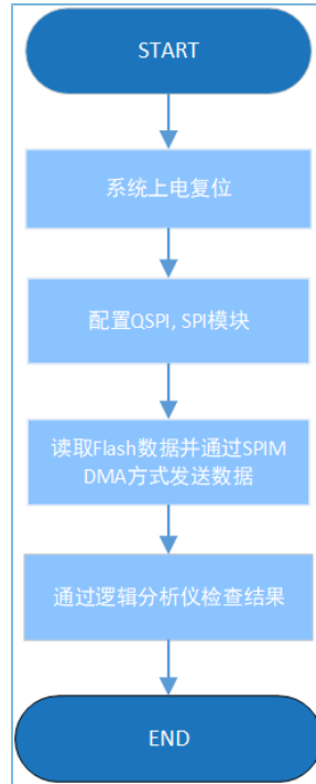
图 3-37 QSPI DMA SPI示例流程图
