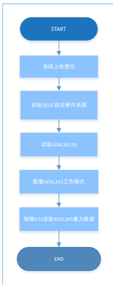
图 3-16 I2C ADXL345示例工程流程图
