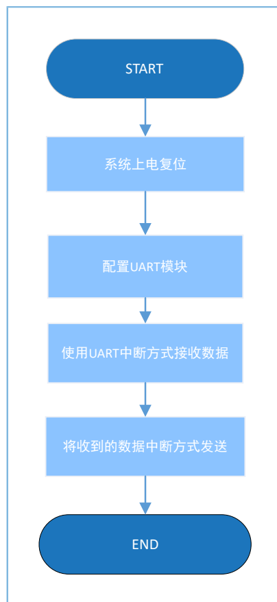
图 3-33 UART Interrupt工程流程图
