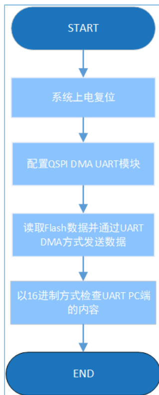
图 3-38 QSPI DMA UART示例流程图
