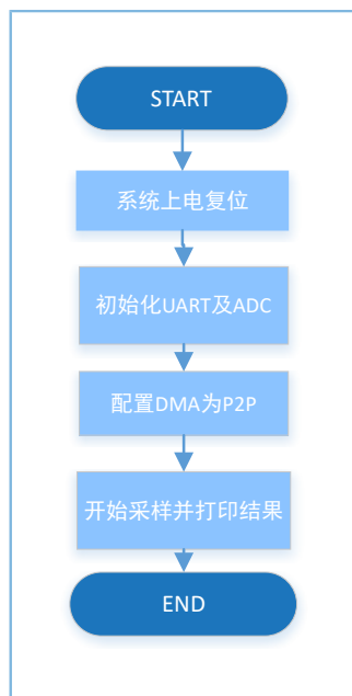
图 3-3 ADC DMA UART示例工程流程图
