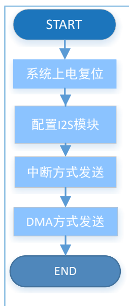
图 3-18 I2S Master Audio 示例工程流程图
