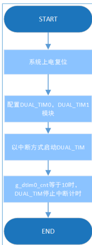
图 3-39 Dual Timer工程流程图
